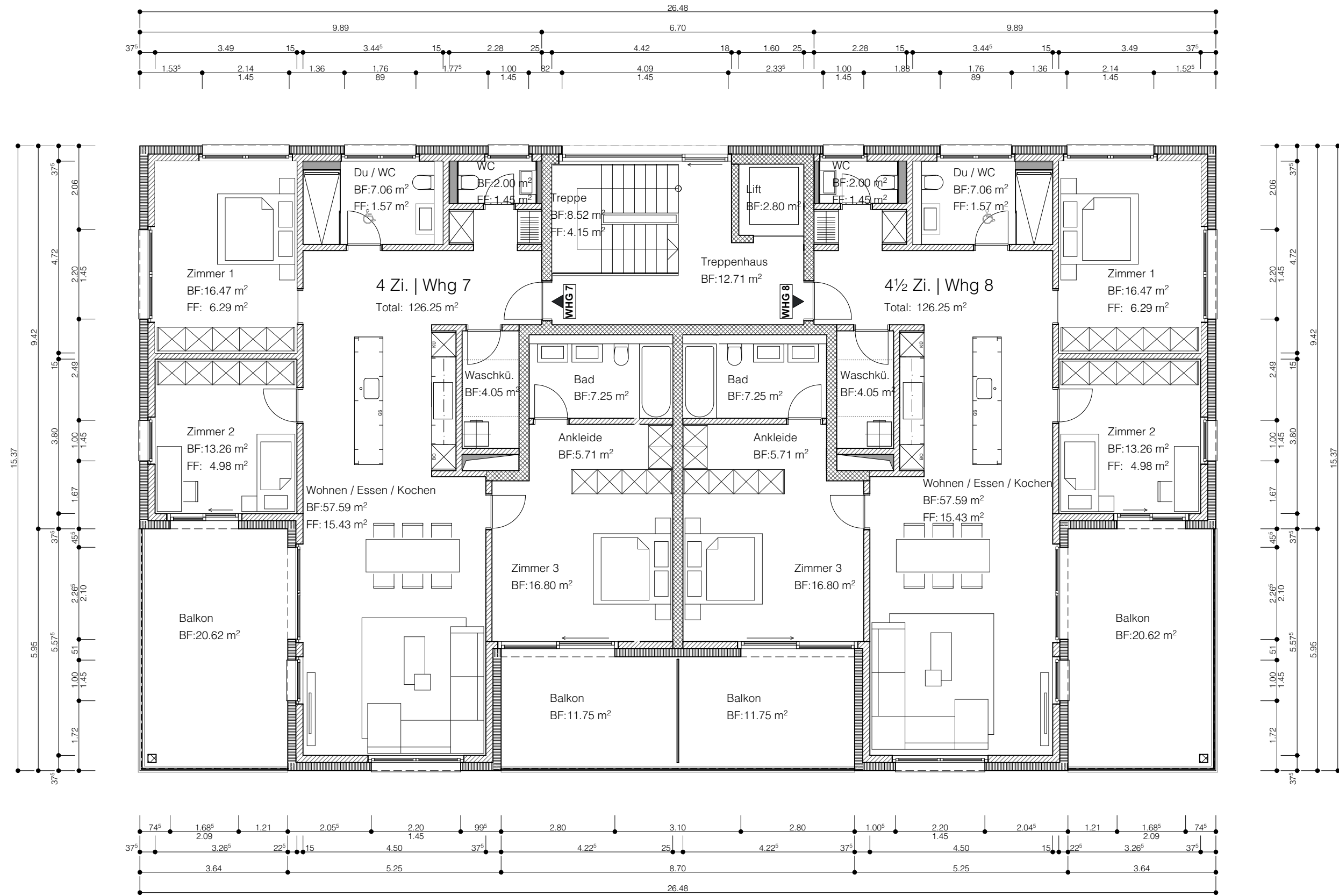
Haus A - 2.Obergeschoss
